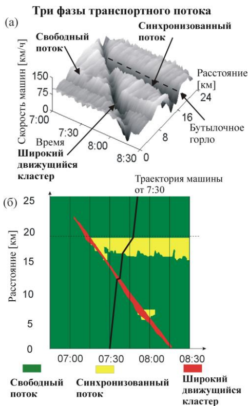
Рис. 3. Данные измерений скорости АТС в пространстве и времени (а) и их представление на координатно-временной плоскости (б). Взято из [1]
