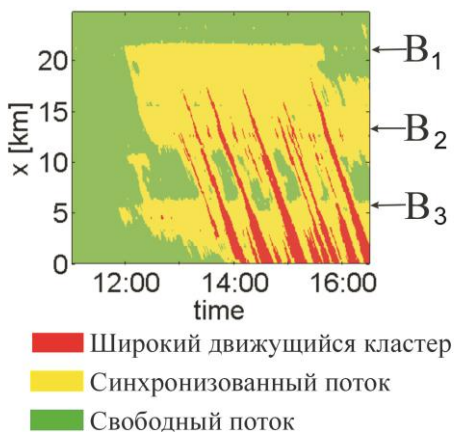
Рис. 11. ЕОП измеренная на магистрали с тремя узкими местами V_1 , V_2 , V_3 . Взято из [1]
