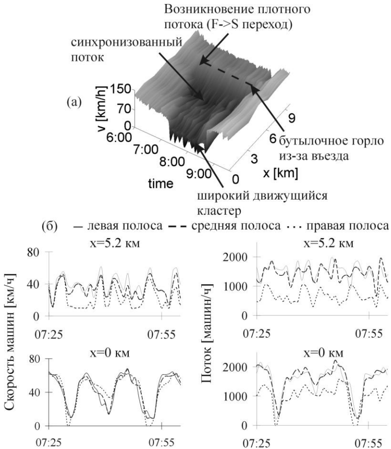
Рис. 5. Эмпирический пример возникновения широких движущихся кластеров в синхронизованном потоке: (а) Скорость АТС в пространстве и времени. (б) Скорость (слева) и поток (справа) на трех полосах дороги в области синхронизованного потока ( x = 5.2 км) и в области широких движущихся кластеров ( x = 0 км). Взято из [1]
