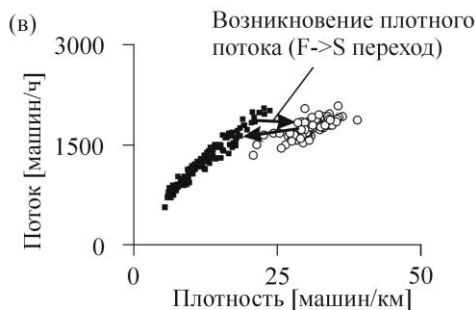
Рис. 4. Эмпирический пример возникновения плотного потока и эффект гистерезиса у бутылочного горла из-за въезда на автодорогу. (а, б) Средняя скорость (а) и поток (б) на автодороге в пространстве и времени (увеличение потока после въезда на (б) связано с потоком въезжающих на дорогу АТС). (в) Эффект гистерезиса в плоскости поток-плотность, обозначенный двумя стрелками, показывающими переход к плотному потоку и обратный переход к свободному потоку. 1-минутные данные. Взято из [1]
