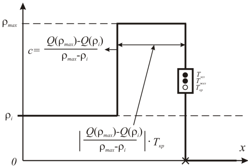
Рис. 22. Момент окончания горения красного цвета
