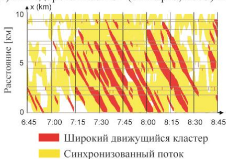
Рис. 15. Пространственно-временная структура транспортного потока, полученная методом ASDA/FOTO в трех странах. Взято из [1]
