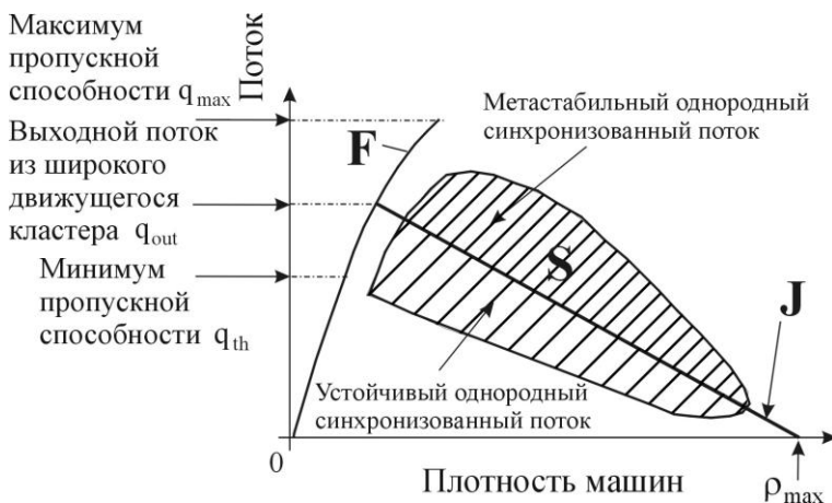
Рис. 9. Три фазы транспортного потока в плоскости поток-плотность в теории трех фаз Кернера. Взято из [1]
