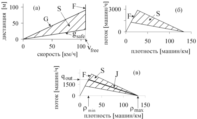
Рис. 12. Стационарные однородные состояния и линия J Кернера в стохастической трехфазной модели: (а, б) свободный поток (F) и синхронизированный поток (заштрихованная двумерная область, обозначенная буквой S) на плоскости расстояние между АТС–скорость (а) и на плоскости поток–плотность (б). На (в) показано соответствие между линией J и однородными стационарными состояниями модели на плоскости поток–плотность, взятыми из (б)
