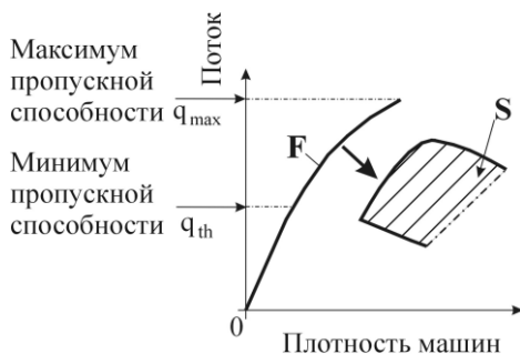
Рис. 7. Максимум и минимум пропускной способности скоростной автомагистрали в теории трех фаз. Взято из [1]
