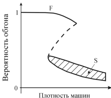
Рис. 6. Объяснение фазового перехода к плотному потоку (traffic breakdown) на основе Z-образной нелинейной функции вероятности обгона (вероятности «переускорения») в теории Б. С. Кернера. Пунктирная линия описывает критическое значение вероятности обгона как функцию плотности АТС (из [1])
