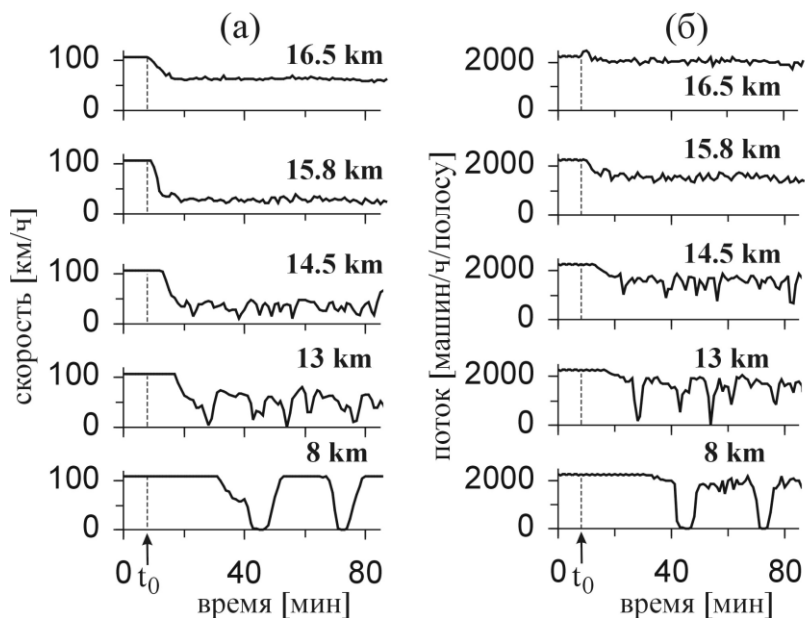
Рис. 14. Одноминутные данные виртуальных детекторов, отвечающие ОП на рис. 13 (д). Въезд на скоростную дорогу отвечает координате 16 км. Взято из [2]
