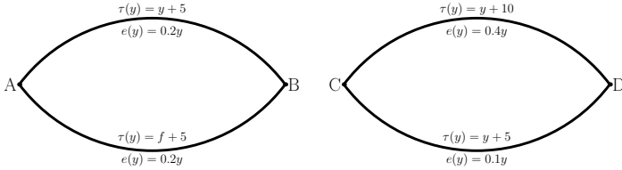
Рис. 6. Сети автомобильных дорог и трамвайных линий
