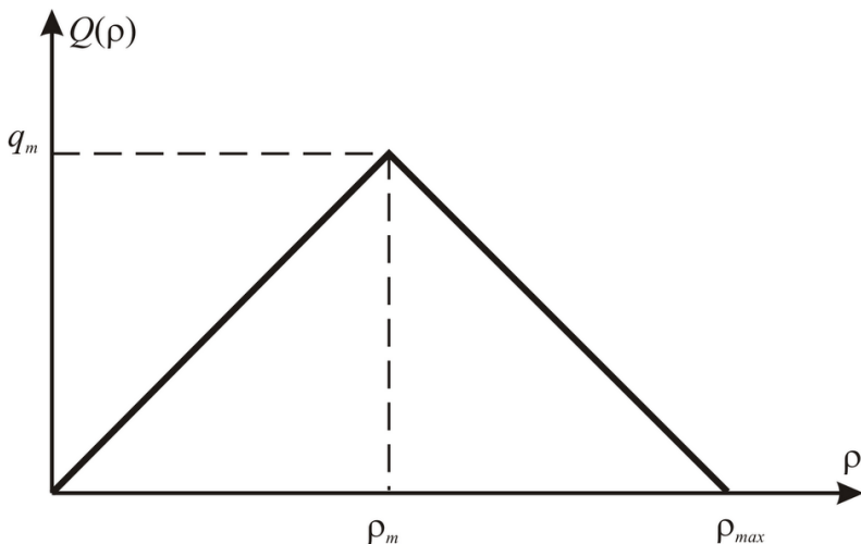
Рис. 8. Треугольная фундаментальная диаграмма
