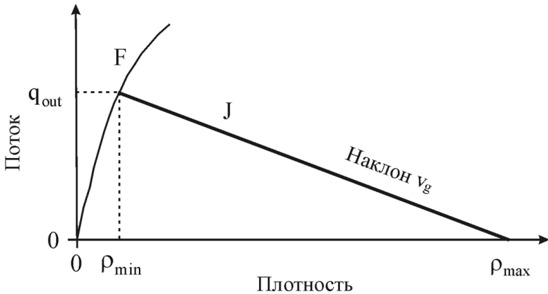
Рис. 28. Качественное представление фундаментальной диаграммы свободного потока (F) вместе с линией J Кернера, наклон которой равен средней скорости движения v_g заднего фронта широкого движущегося кластера. Взято из [10]
