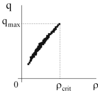
Рис. 1. Зависимость потока q от плотности АТС \rho в свободном потоке [14, 20]
