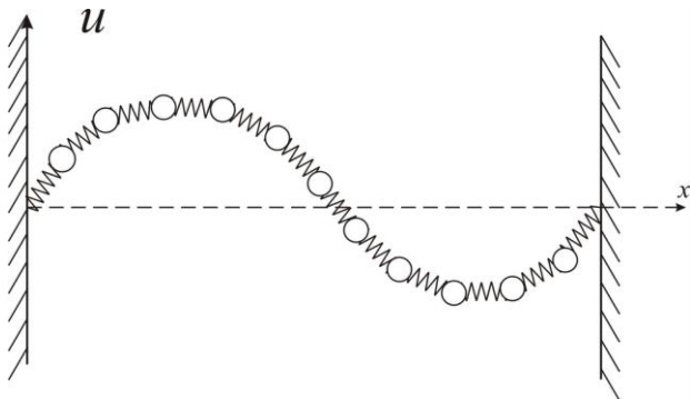
Рис. 10. Колебания струны, Д'Аламбер (1780)
