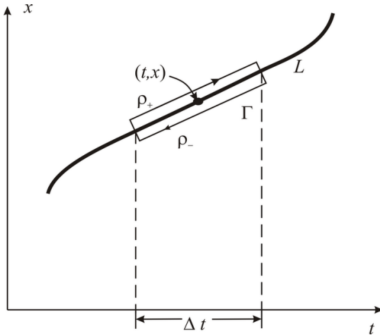
Рис. 3. RRH-условие на разрыве
