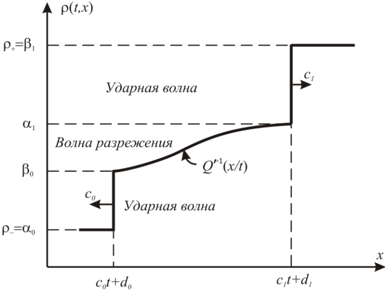
Рис. 18. Система волн
