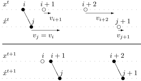
Рис. 2. Спаривание частиц. Взаимно спаренные частицы обозначены черными кружками и соединены прямыми линиями, а дефекты — белыми кружками. В момент t частицы i и j спарены, тогда как в момент t + 1 x -частица i становится неспаренной, а \hat{x} -частица j спаривается с x -частицей i + 1 . Неспаренные в момент t частицы i + 2 и j + 1 спариваются в момент t + 1
