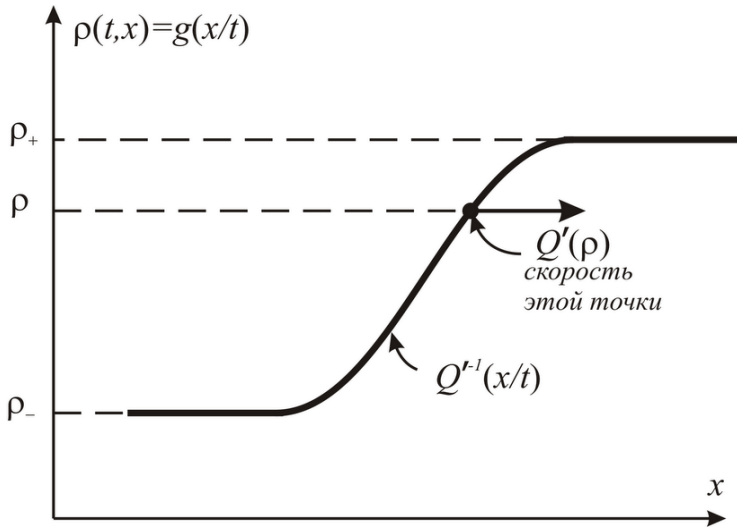
Рис. 16. Волна разрежения
