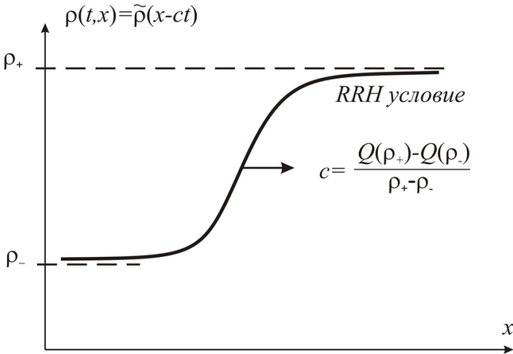
Рис. 19. Бегущая волна
