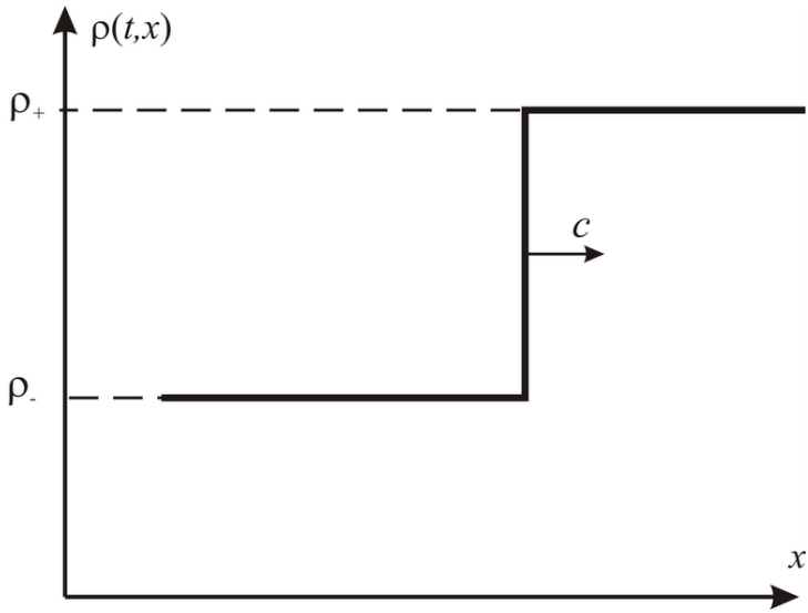
Рис. 15 Ударная волна
