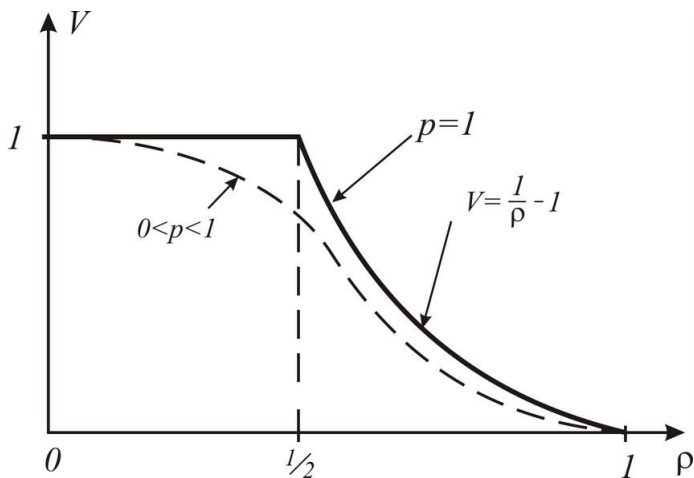
Рис. 11. «Фазовый переход» при \rho = 1/2
