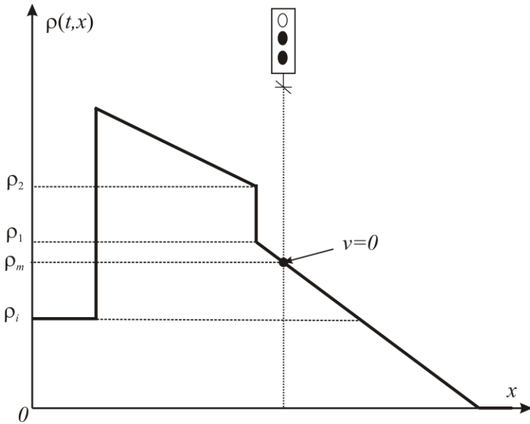
Рис. 24. Горит зеленый цвет
