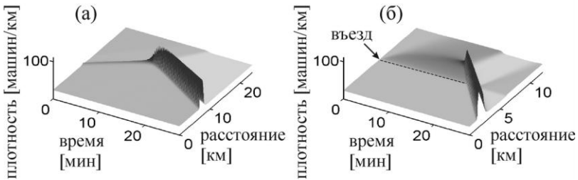
Рис. 25. Эффект «бумеранга» для нарастающего возмущения в свободном потоке, метастабильном относительно возникновения широких движущихся кластеров. Плотность АТС в пространстве и времени. Расчет на основе макроскопической модели Пэйн-класса (22), (23). (а) Однородная автодорога, (б) автодорога с въездом. Взято из [10]
