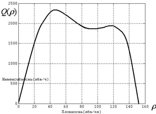
Рис. 2. Фундаментальная диаграмма
