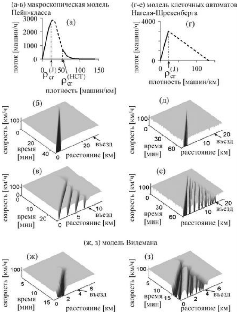
Рис. 26. Возникновение плотного потока на автодороге с въездом в моделях ДМ-класса, показывающих неустойчивость свободного потока при повышении плотности: возникновение широких движущихся кластеров в макроскопической модели (10), (11) Пэйн-класса (а-в), в модели клеточных автоматов Нагеля-Шрекенберга (г-е), и в модели Видемана (ж-з). (а, г) Фундаментальная диаграмма в макроскопической модели Пэйн-класса (а) и в модели Нагеля-Шрекенберга (г); пунктирная часть диаграмм отвечает неустойчивым состояниям. (б, в, д-з) Средняя скорость АТС в пространстве и времени. Взято из [10]
