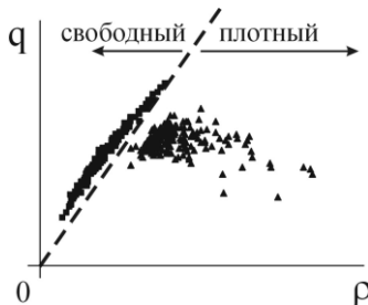
Рис. 2. Зависимость потока от плотности АТС в свободном и плотном потоке [14, 20]
