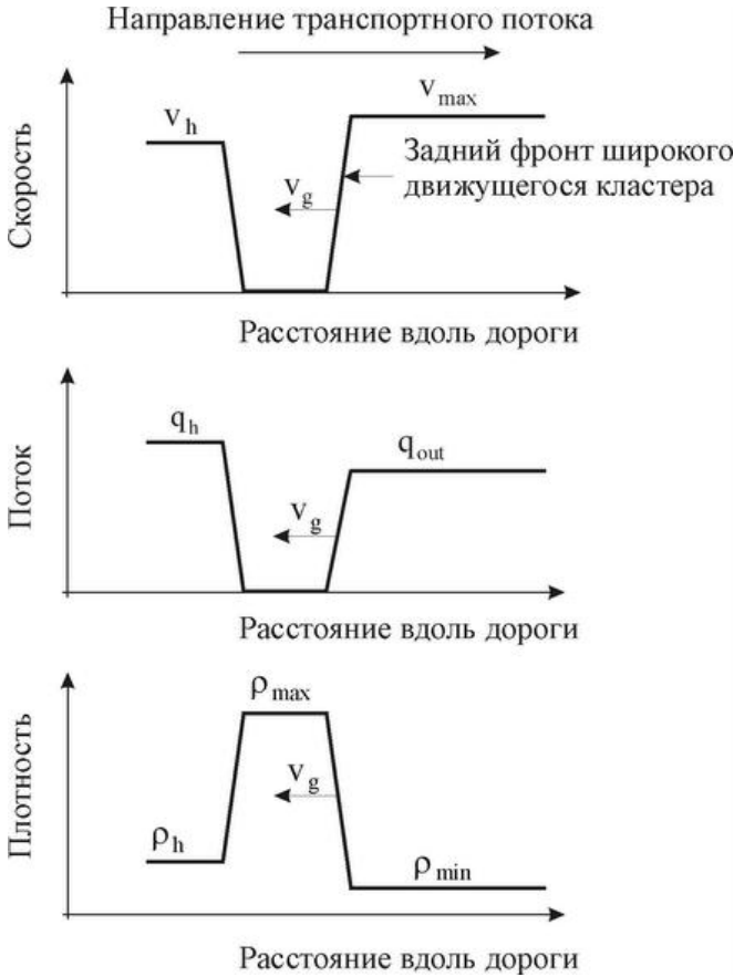
Рис. 27. Качественная иллюстрация характеристических параметров широкого движущегося кластера. Схематическое представление кластера в фиксированный момент времени. Пространственные распределения скорости АТС v , потока q , и плотности \rho в широком движущемся кластере, который распространяется в исходно однородном свободном потоке, имеющем скорость v_h , величину потока q_h , и плотность \rho_h . Взято из [10]
