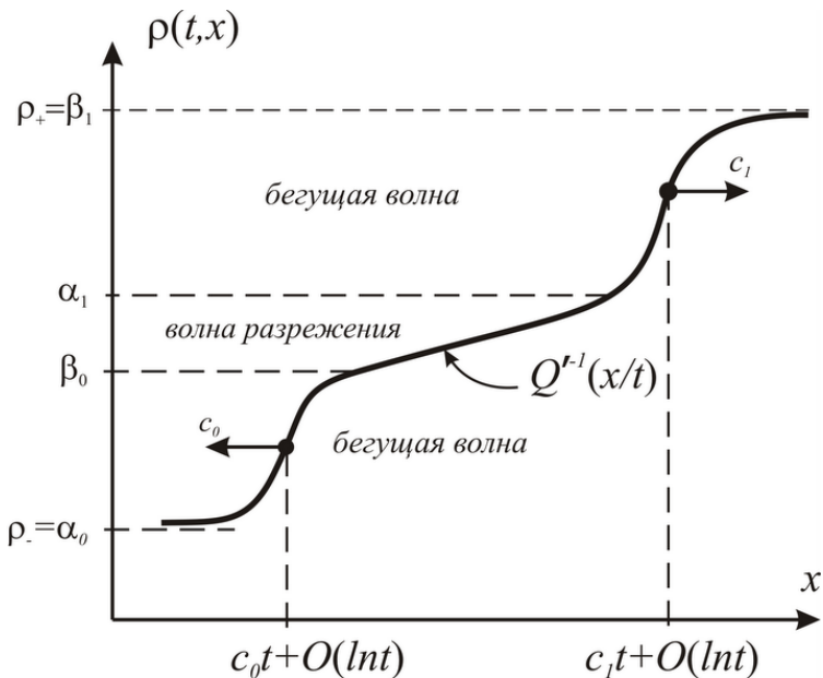
Рис. 20. Система волн
