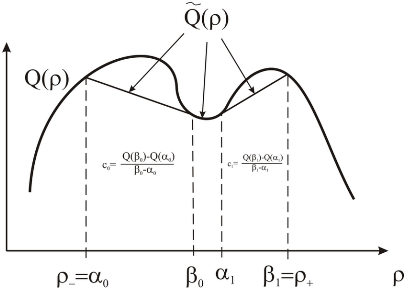
Рис. 17. Построение И. М. Гельфанда (1958)
