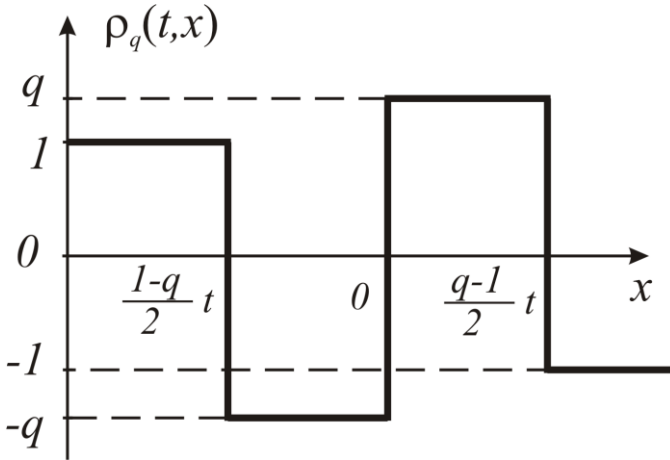
Рис. 4. Пример О. А. Олейник (1957)
