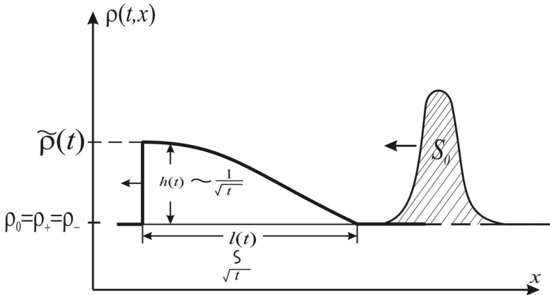
Рис. 21. Эволюция локального затора
