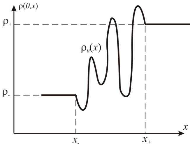
Рис. 14. Начальное условие типа Римана
