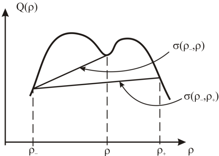
Рис. 5. E-условие
