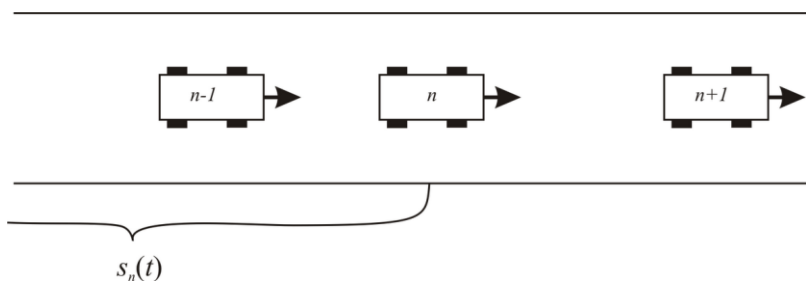
Рис. 9. Микроскопическая модель
