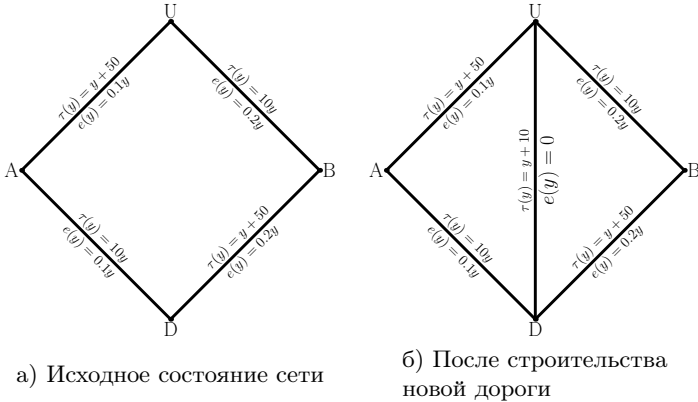
Рис. 3. Парадокс Брайеса
