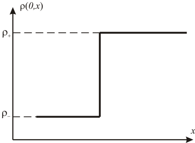
Рис. 13. Начальное условие Римана
