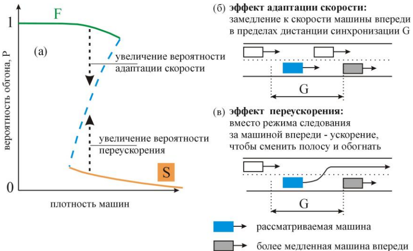
Рис. 8. Пояснение соревнования между переускорением и адаптацией скорости, которое объясняет бесконечное число значений пропускной способности автомагистрали. Взято из [1]
