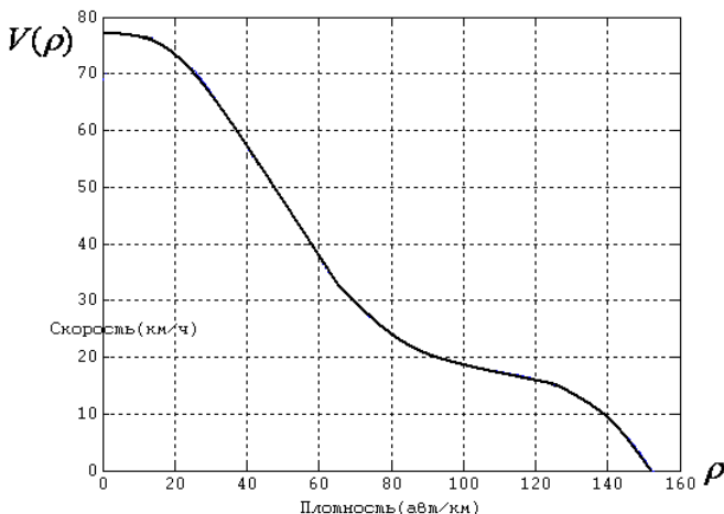
Рис. 1. Уравнение состояния транспортного потока
